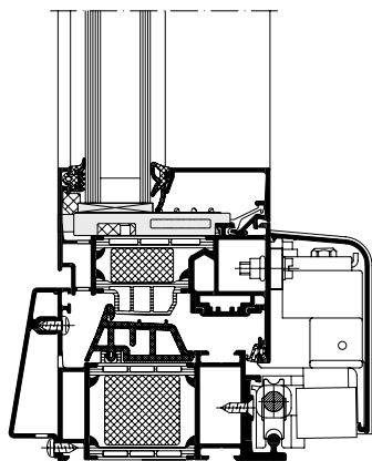
Elemento PASK con automatismo Tilt/slide unit with engagement mechanism
